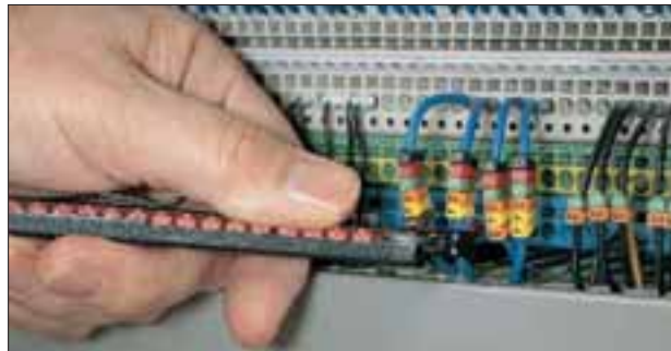
Benytt WIC-tool for enkelt å sneppe merkingen på kabelen.
