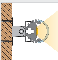
Schwenkhalter für Boden- oder Wandmontage swiveling holder for floor and wall mounting
