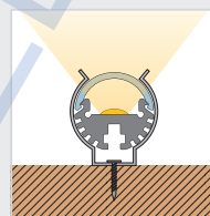
Montage mit Halteklammer mounting with clips
