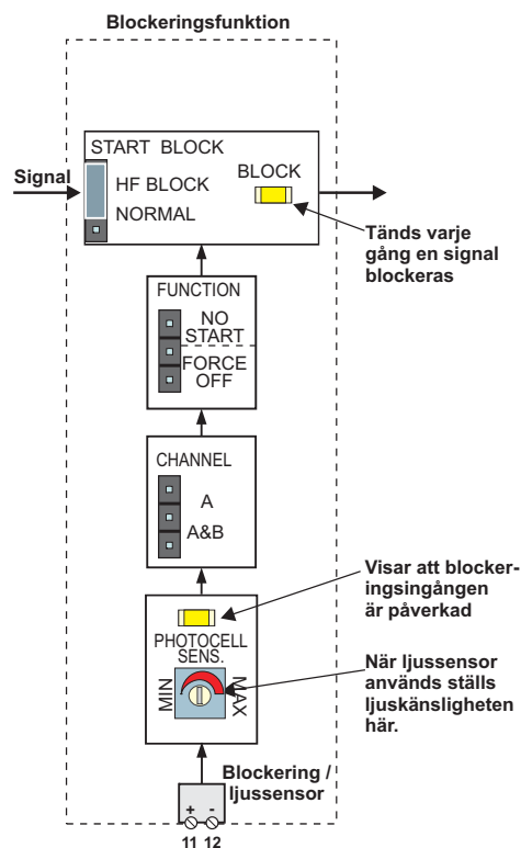
Blockeringsfunktionens principiella uppbyggnad.
