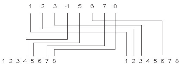
SPLITTLEDD TELE/DATA LAN 23
