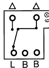
Koblingskjema
