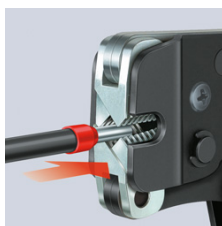
Frontal innføring av lederendehylser f.eks i koplingskap
