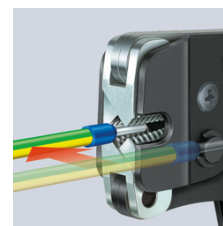
97 53 08 innføring av lederendehylser parallelt fra siden inntil 2,5 mm 2 f.eks under trange plassforhold
