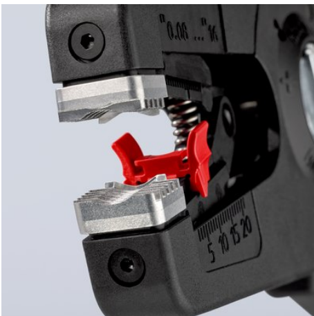
Halvsirkelformet, rillet holdeklemme for bedre grep som holder så godt som all isolasjon sikkert på plass
