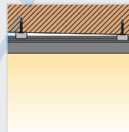
Ausgleich unebener Decken und Wände durch drei Profilarretierungen equilization of uneven ceilings and walls by three profile rockings
