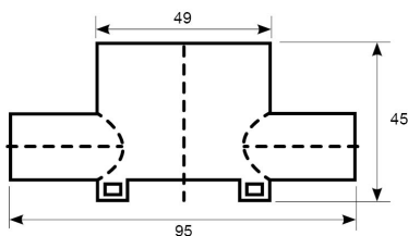
Målskisse
