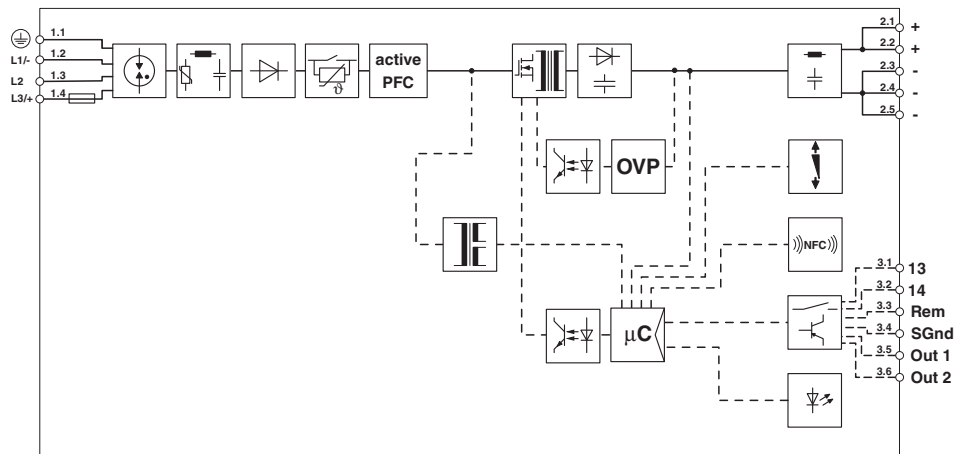
Blokkskjema
