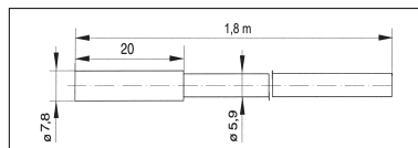
Temperaturgivarens mått
