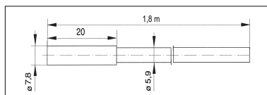
Dimensioni della sonda
