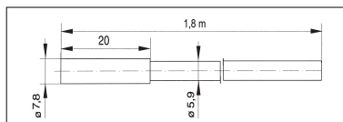
Maße des Fühlers
