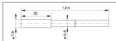
Afmetingen van de sensor
