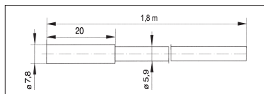
センサーの寸法
