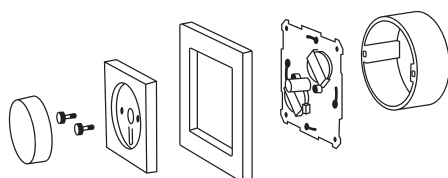
Montering utenpå veggbokser.
