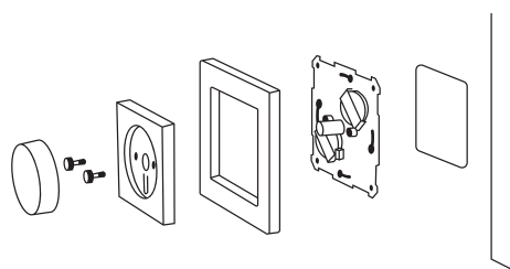
Montering med medfølgende tape på vegg/flis.
