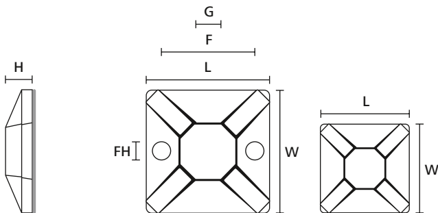
Festesokkel MB3 - MB5 (sett fra siden)
