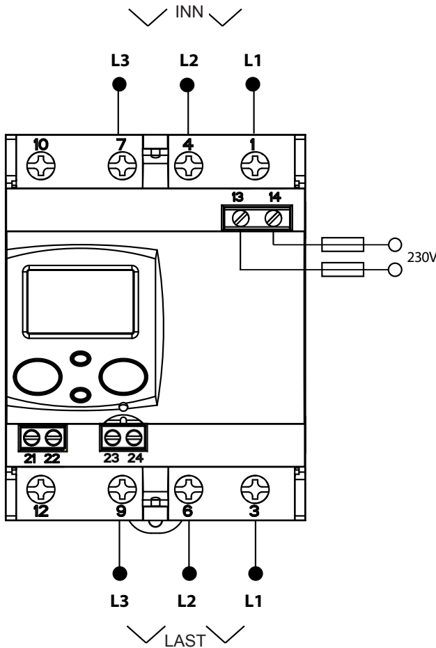
Koblingsskjema 230 V, SE-C21-RS485
