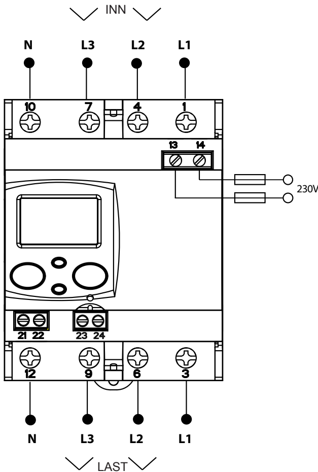
Koblingsskjema 400 V, SE-C21-RS485
