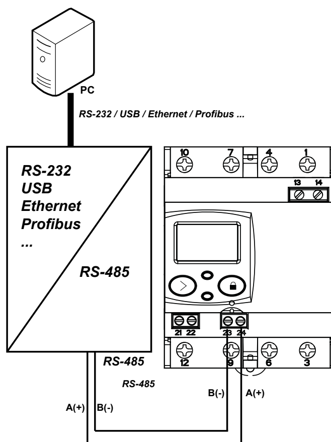
Figur 18: SE-C21-485-T1 og SE-C21-485-DS koblingsdiagram.
