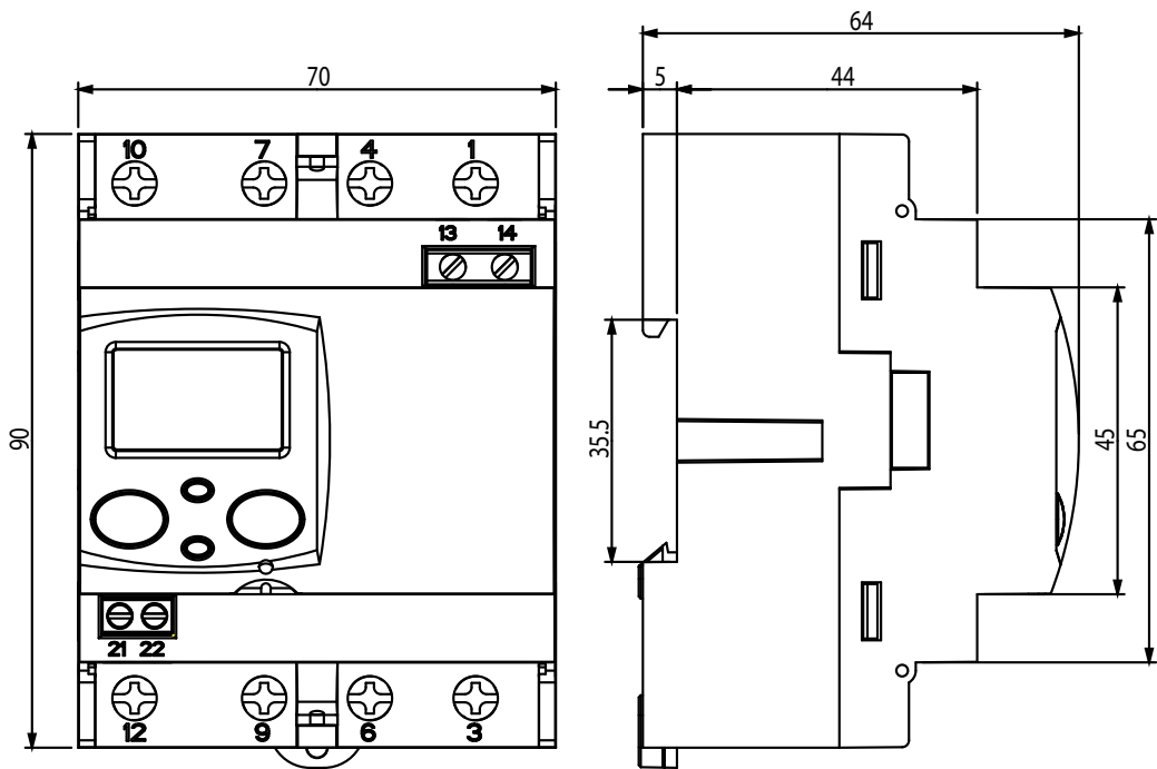
Figur 19: Dimensjoner SE-C21
