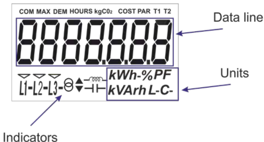
Figure 7: Skjermområder på SE-C20
