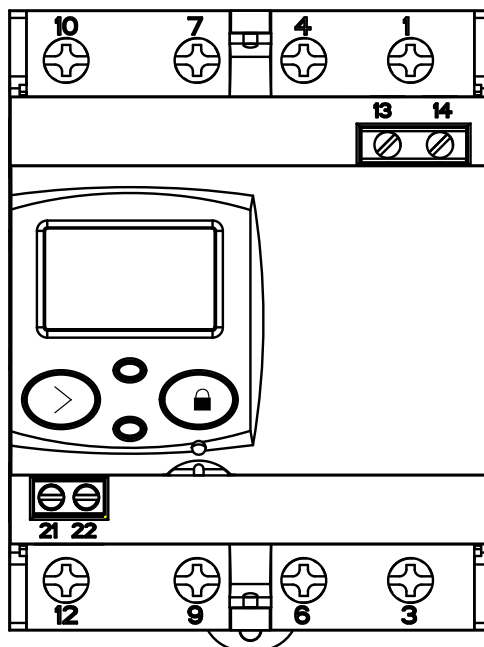
Figur 1:Terminalene på SE-C21-T1.
