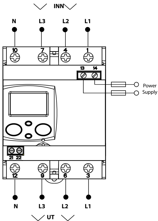
Figur 3: Koblingsskjema SE-C21
