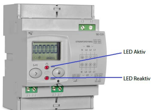
Figur 8: LED Indikatorer på SE-C21
