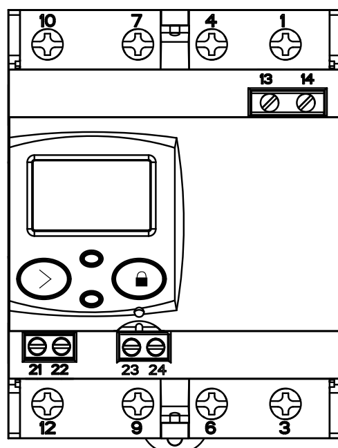
Figur 2: Terminalene på SE-C21-485-T1 and SE-C21-485-DS.
