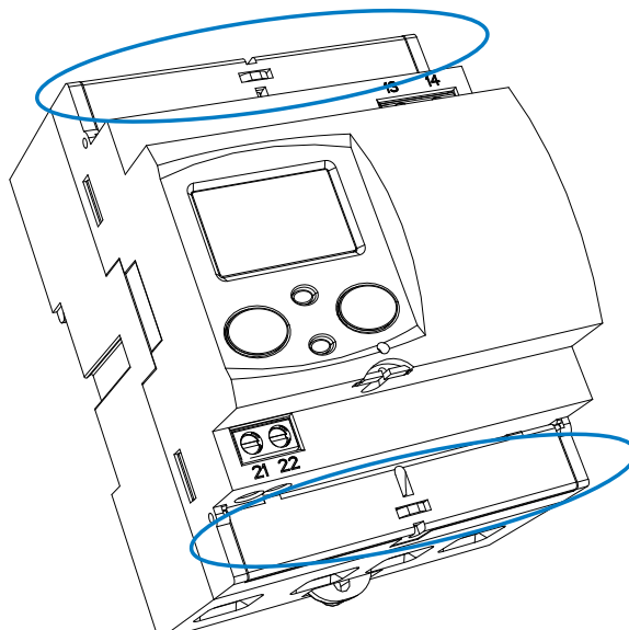
Figur 4: Terminaldeksler på SE-C21
