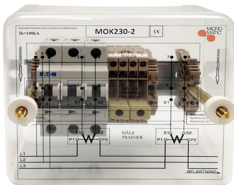
Bilde viser MOK 230V El.nr 8200100
