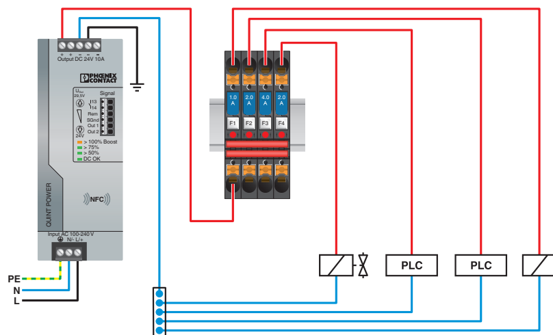
Applikasjonstegning
