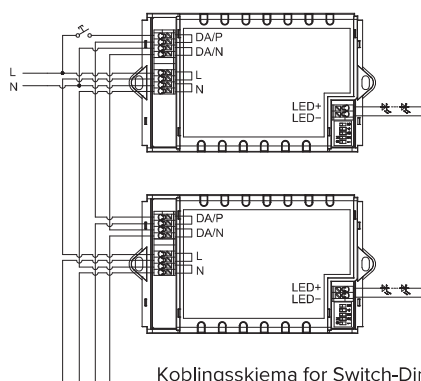
Koblingskjema for Switch-Dim
