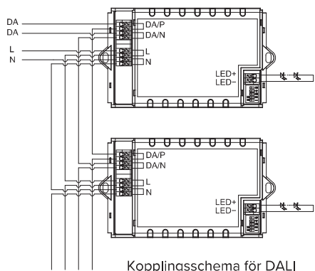
Kopplingschema för DALI
