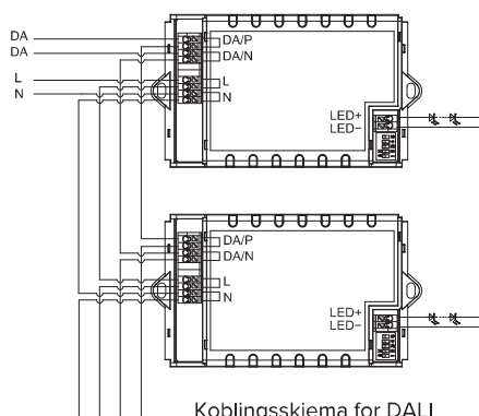
Koblingskjema for DALI
