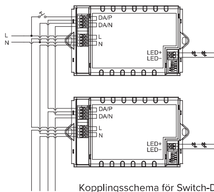
Kopplingschema för Switch-Dim
