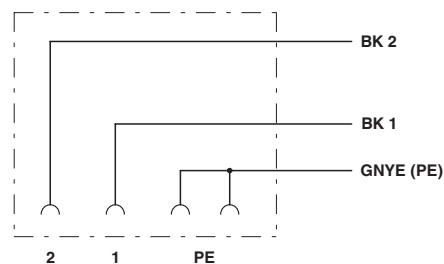
Koblingsskjema
