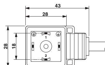
Målskisse
