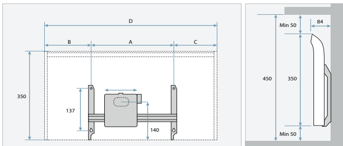
Mål: Glamox 3001 TPA Høy
