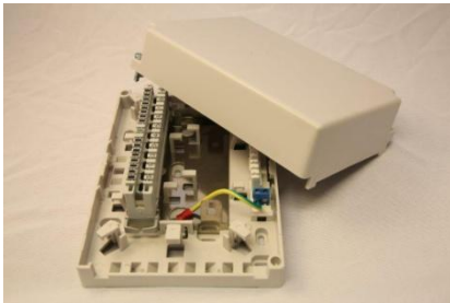
10 par m/plass for ekstra 10 par plint
