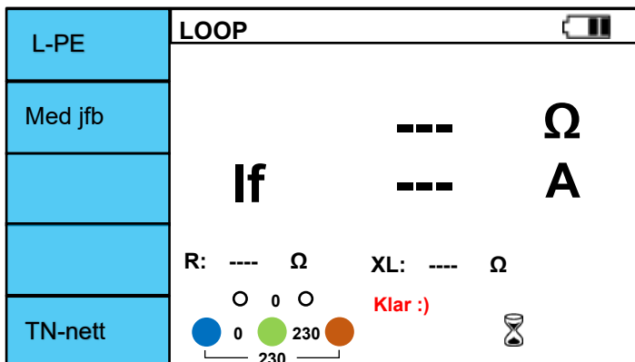
Figure 6.5.2 Bryter og skjerm før måling
