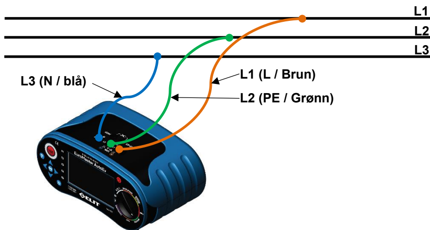
Figure 6.4.4 Tilkobling dreieretningsmåling
