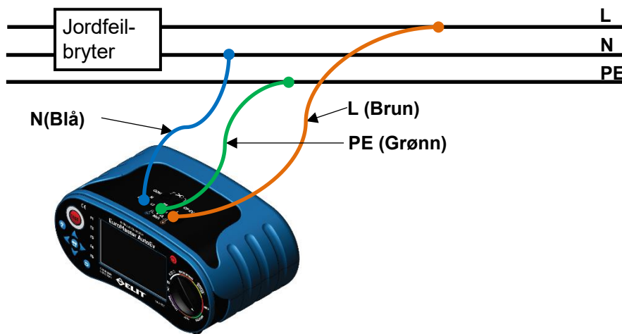
Figur 6.5.1 Tilkobling Z-sløyfe med jordfeilbryter ELIT PC-2 pluggadapter kan også benyttes
