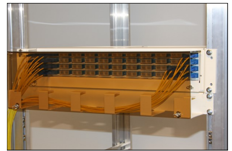
Panel med kabelrenne og deksel i FR70 stativ
