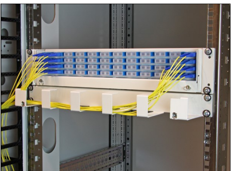
Panel med kabelrenne i standard 19" skap
