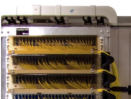
Rack med panel og toppkanal
