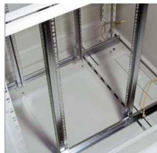
Fleksiramme for kombinert 19"/21" og sideforskyvning
