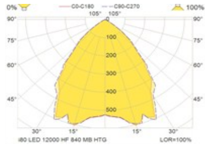
i80 Medium strålevarmetestet herdet glass (HTG)
